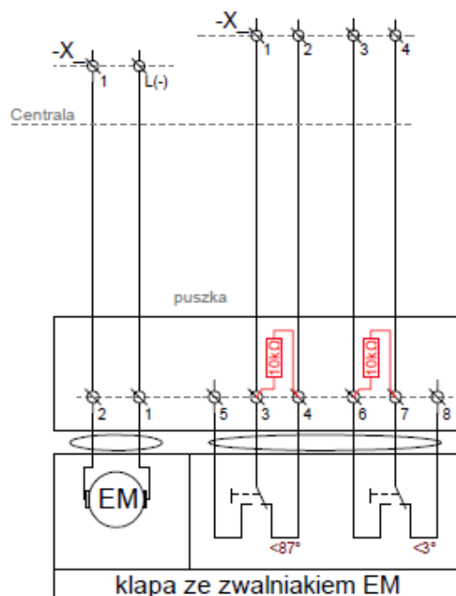
Rys. 21. Schemat siłownik ze zwalniającym.
